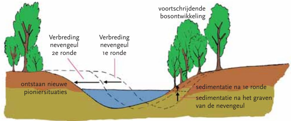
Fig. 2. Het principe van een verschuivende nevengeul, waarbij op de ene oever steeds nieuwe pioniersituaties ontstaan, terwijl op de andere oever de ontwikkeling ongestoord door kan gaan.
