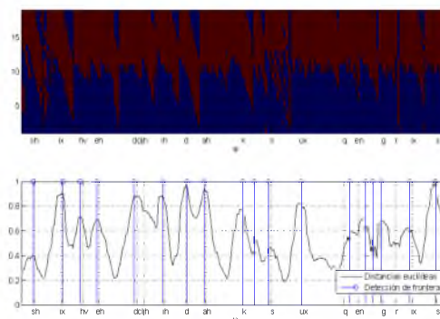
Figura 4. a) Representación del agrupamiento por ventanas en un segmento de voz. b) Representación de las distancias euclídeas entre clases para el mismo segmento de voz que a) y segmentos detectados aplicando un método de detección de mínimos locales.
