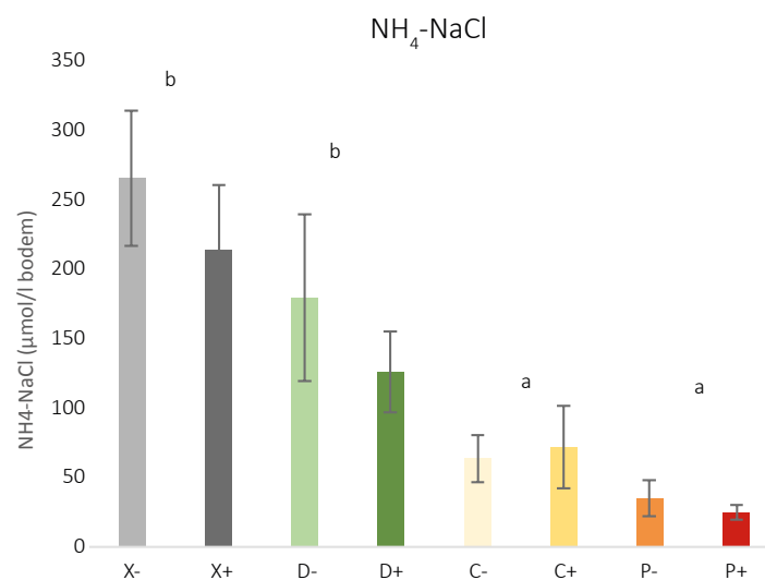
Fig. 2. Gemiddelde concentratie uitwisselbaar ammonium ( \pm standaardfout) na zes jaar in de bodem bij de verschillende maatregelen. X = controle, D = drukbegrazing, C = chopperen en P = pluggen, - = zonder bekalking, + = met bekalking. Foutbalken geven de standaardfout weer. Letters geven de significante verschillen ( p < 0,05 ) tussen behandelingen aan, waarbij de betreffende maatregel met en zonder bekalking samen is getoetst. Er waren geen interactie-effecten tussen kalk en de maatregelen.
